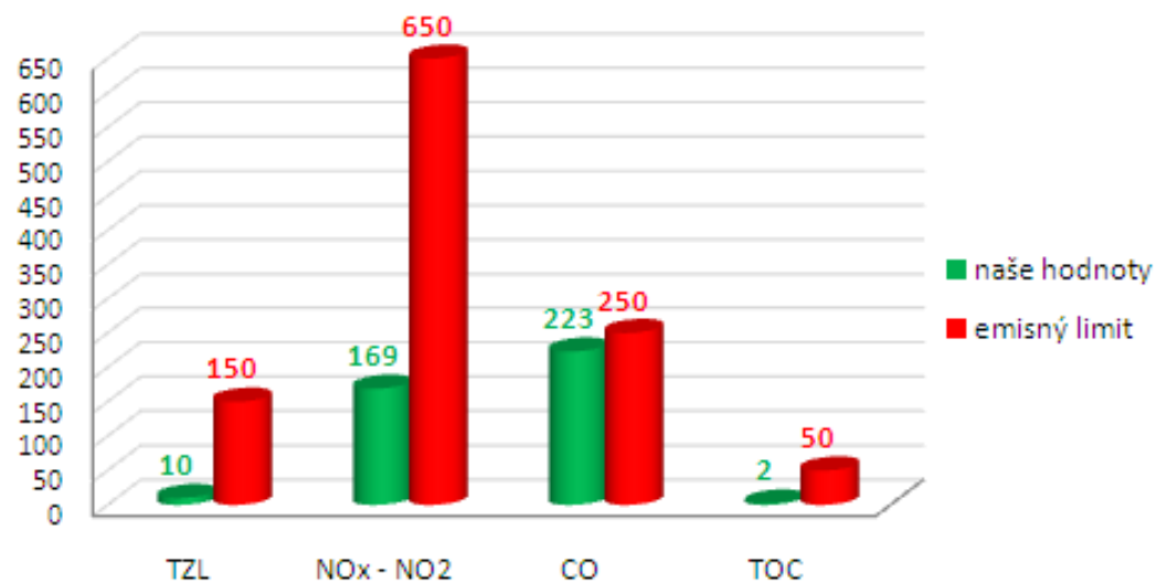
Meranie emisií - kotolňa na biomasu
