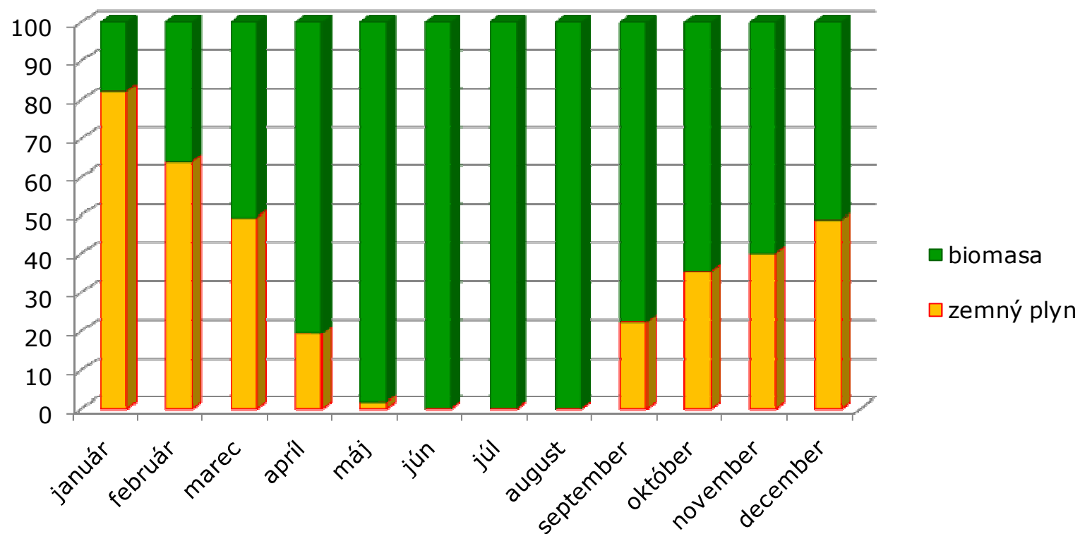
Percentuálny pomer výroby tepla v roku 2011 biomasa/plyn
