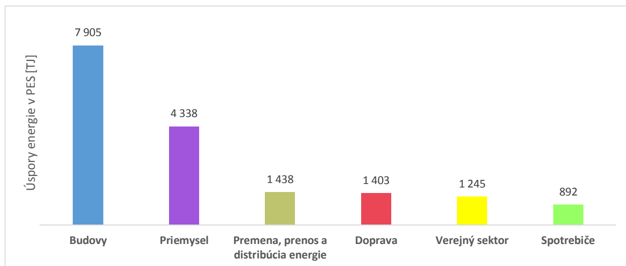
Graf 2: Dosiahnuté úspory energie vo forme PES za roky 2014-2016 [TJ]
